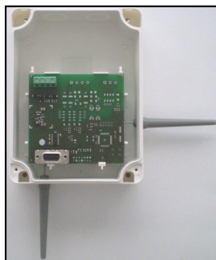
Figura 2 - Panoramica interna del modulo espansore
