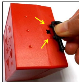
Figura 10 - rimozione del blocco frontale dal supporto di installazione a parete
